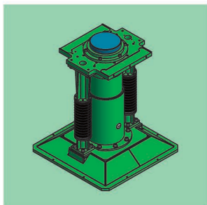
PIATTELLO / PLATE / ASSIETTE (750X 750 MM) 30ton
