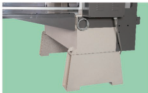
LA MACCHINA È DOTATA DI PIEDI REMOVIBILI PER RIDURRE L'ALTEZZA MASSIMA PER IL TRASPORTO THE MACHINE IS EQUIPPED WITH REMOVABLE FEET TO REDUCE THE MAXIMUM HEIGHT FOR TRANSPORTATION MACHINE EST ÉQUIPÉE DE PIEDS AMOVIBLES POUR RÉDUIRE LA HAUTEUR MAXIMALE POUR LE TRANSPORT
